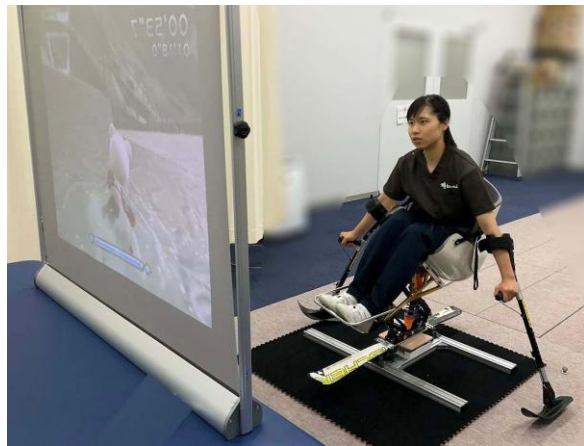
チェアスキーシミュレーター ※神奈川リハ病院 開発
